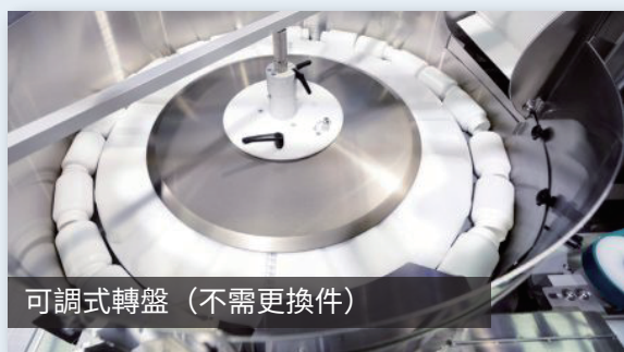
排瓶系統
