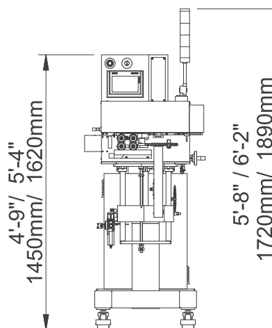
正視圖
